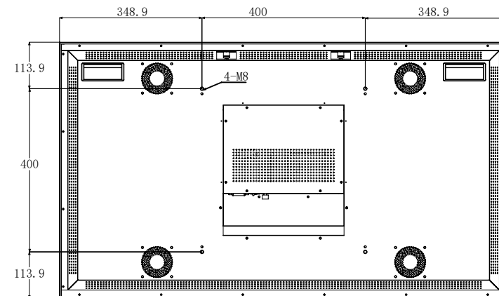
SV-WFD490W HB Dimensiones en mm
