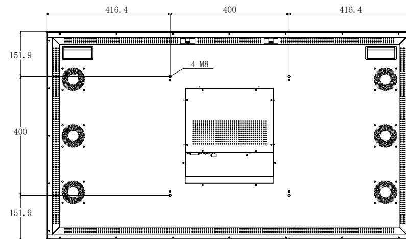
SV-WFD550W HB Dimensiones en mm
