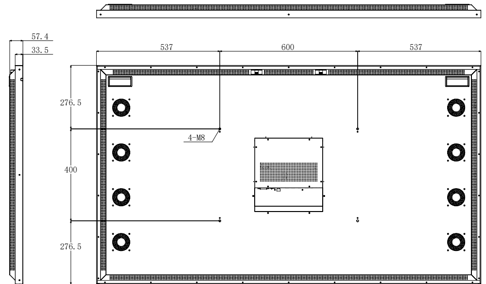
SV-WFD750W HB Dimensiones en mm
